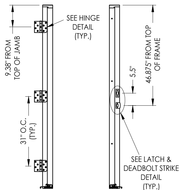
HINGE JAMB STRIKE JAMB
